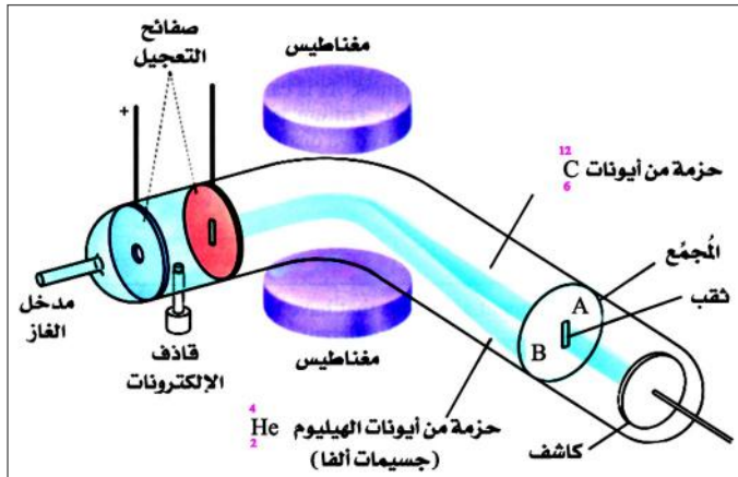
شكل (١-٤) مطياف الكتلة
