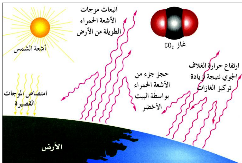
شكل (٢-٩) ظاهرة الاحتباس الحراري
