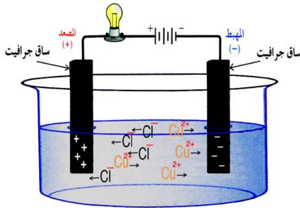
شكل (٣-١١) التحليل الكهربى لمحلول \text{CuCl}_2
