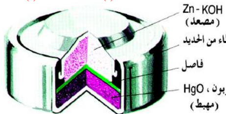
شكل (٨-٣) خلية الزئبق
