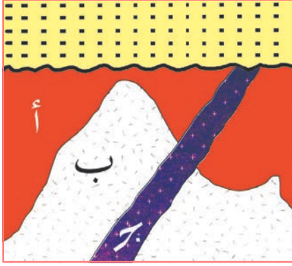
الشكل (٢٤) القاطع أحدث من المقطوع
