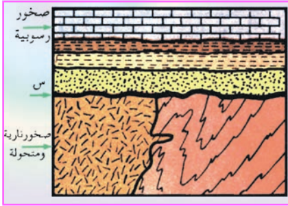
الشكل (٥) عدم التوافق المتباين
