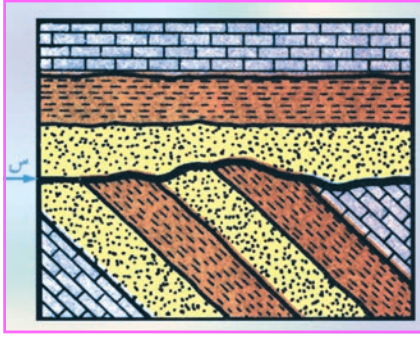
الشكل (٤) عدم التوافق الزاوي
