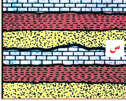
الشكل (٣) عدم التوافق الحثي
